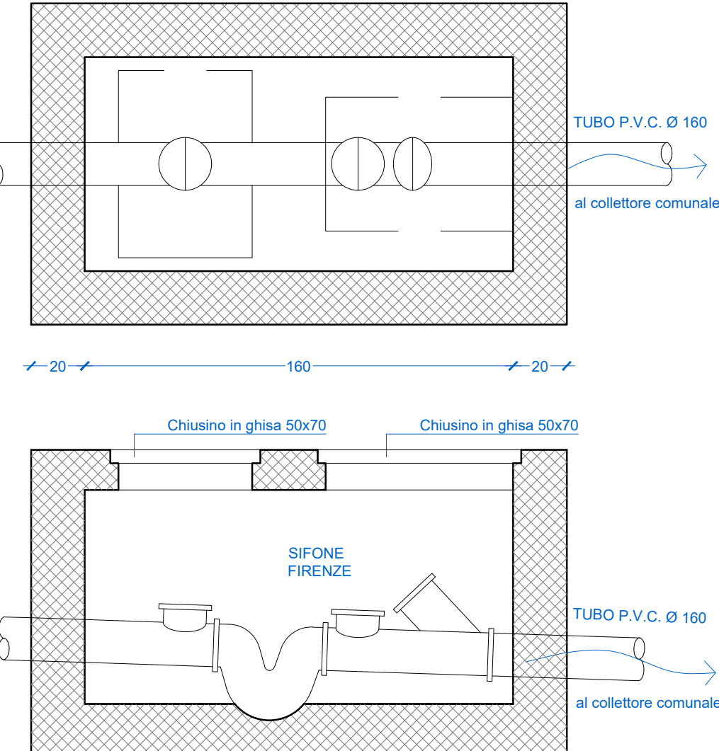
PARTICOLARE POZZETTO DI ISPEZIONE SIFONE FIRENZE Scala 1:20
