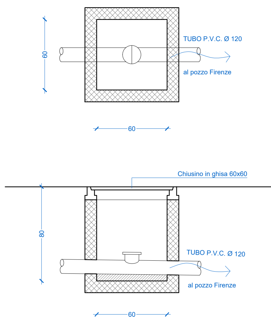
PARTICOLARE POZZETTO DI ISPEZIONE - PN01 Scala 1:20
