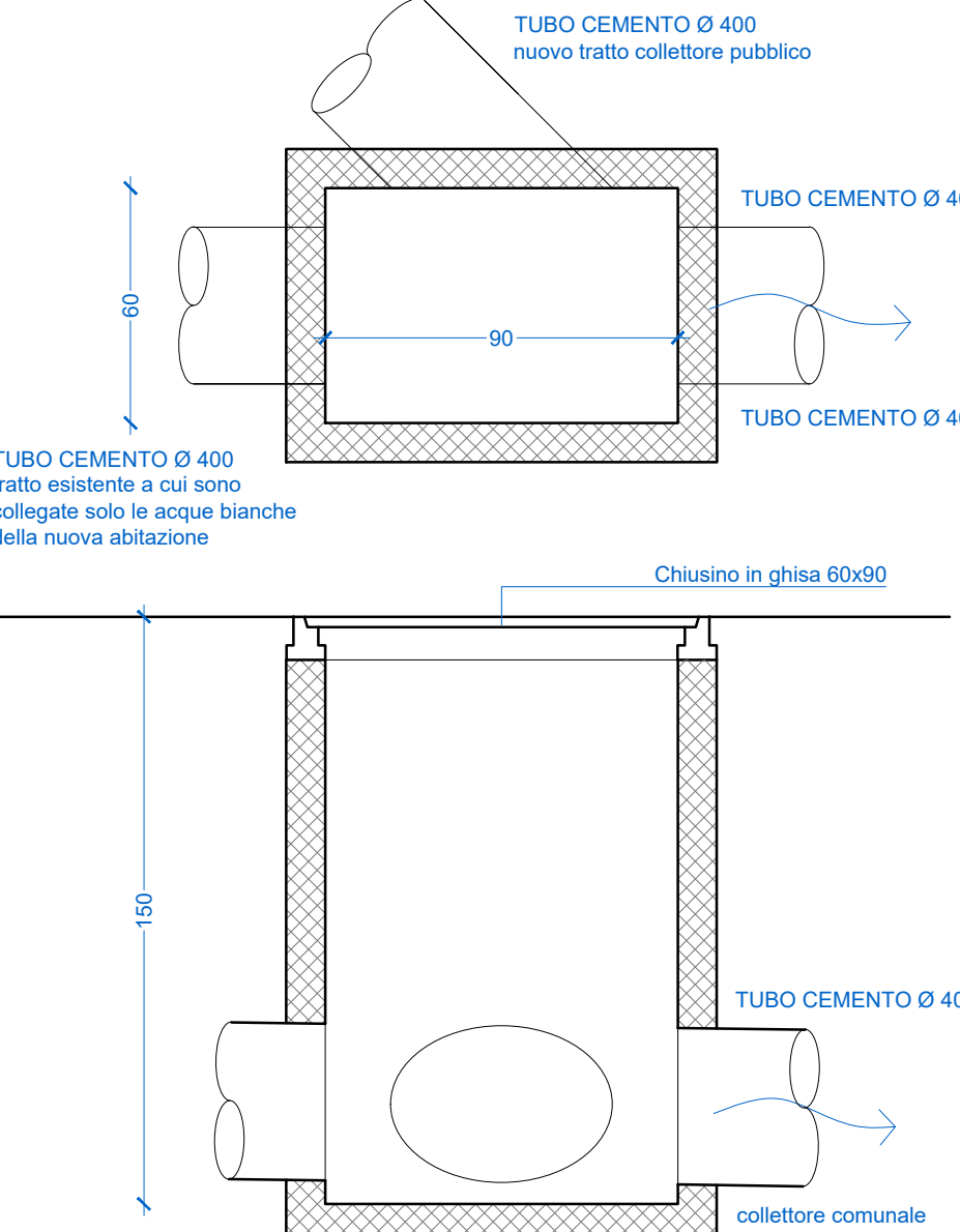
PARTICOLARE POZZETTO ISPEZIONE ACQUE BIANCHE - PBP03 Scala 1:20
