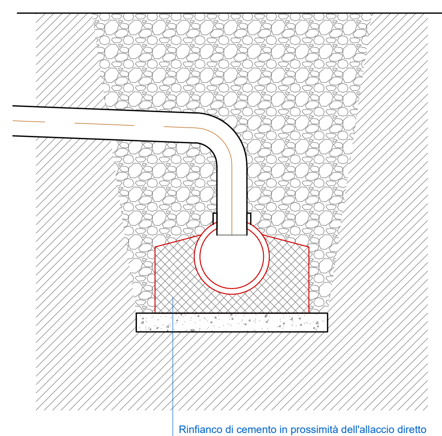
PARTICOLARE ALLACCIAMENTO DIRETTO AL COLLETTORE Scala 1:20
