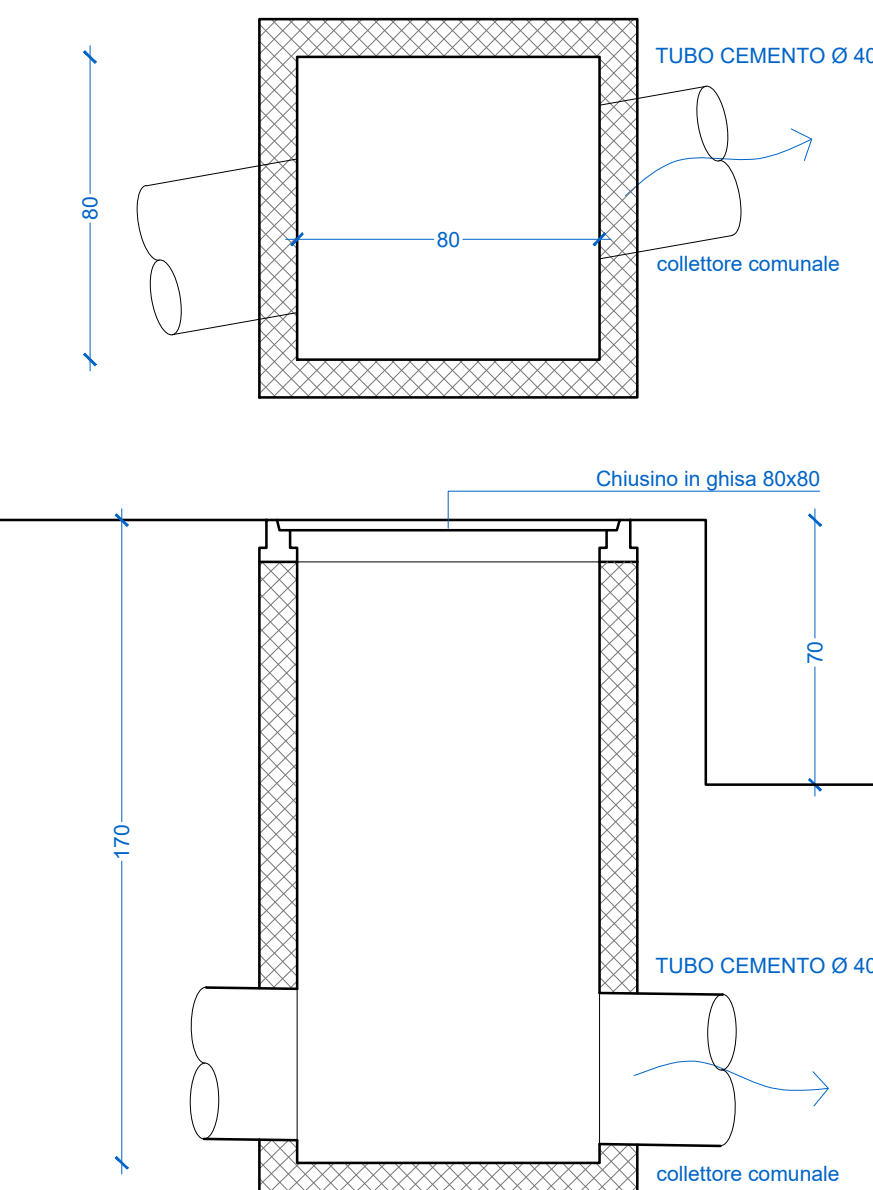
PARTICOLARE POZZETTO ISPEZIONE ACQUE BIANCHE - PBP01 Scala 1:20
