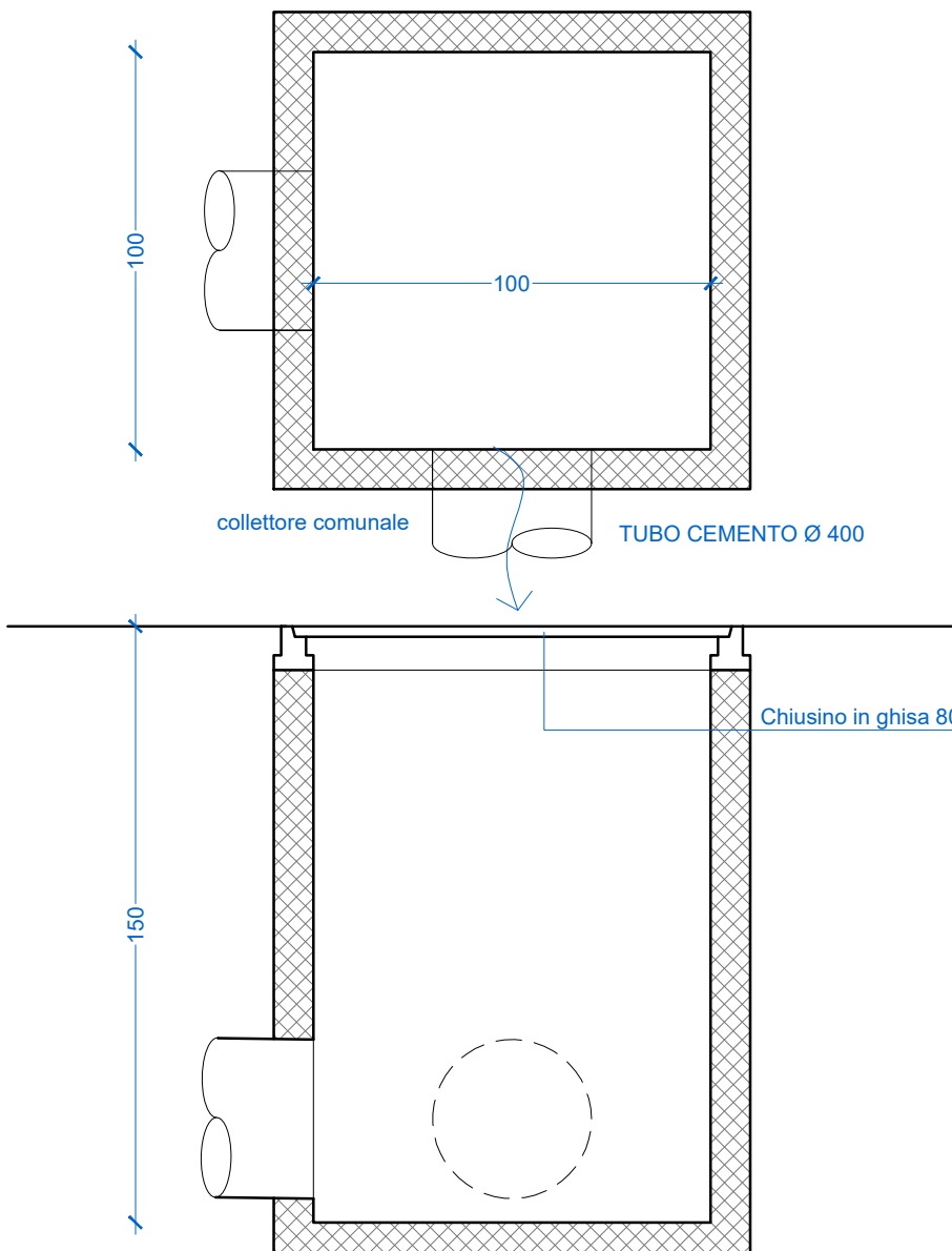
PARTICOLARE POZZETTO ISPEZIONE ACQUE BIANCHE - PBP02 Scala 1:20
